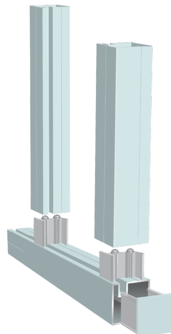
Kaide jakoprofiili, uran syvyys 15 mm
