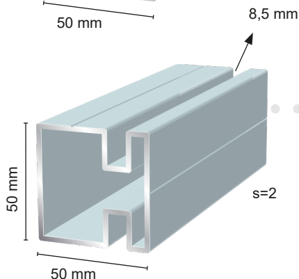
Kaide jakoprofiili, uran syvyys 15 mm
